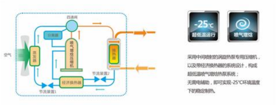
超低温喷气增焓热泵的系统示意图
